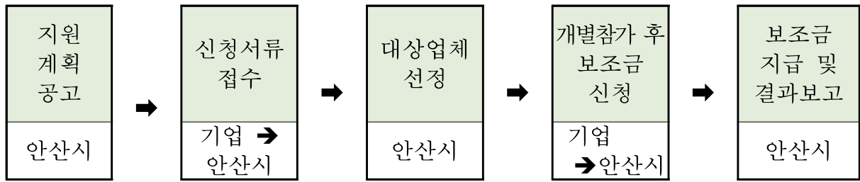
<사업추진 흐름도>
